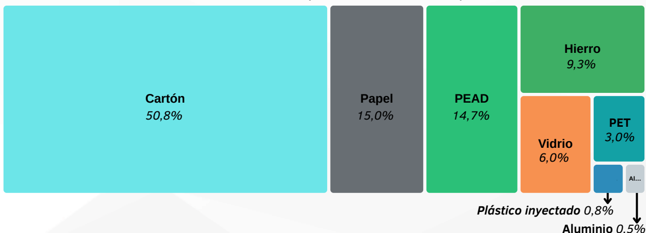
Figura 7: Cantidad de materiales reciclables (en kilogramos) recibido en el centro de acopio. Acumulado anual (enero a octubre 2024).
